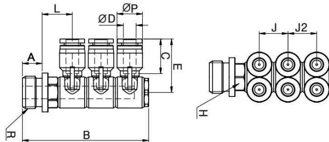
Размери / Dimension Chart
